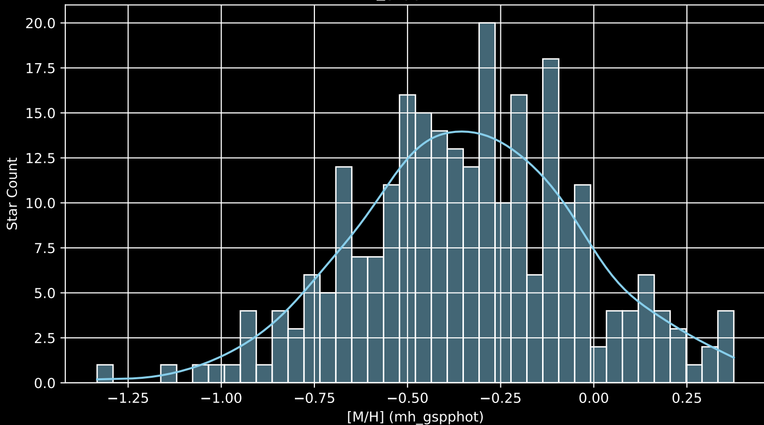
GALAH DR4 Field: [350] [M/H] (mh_gspphot) (n= 256)
