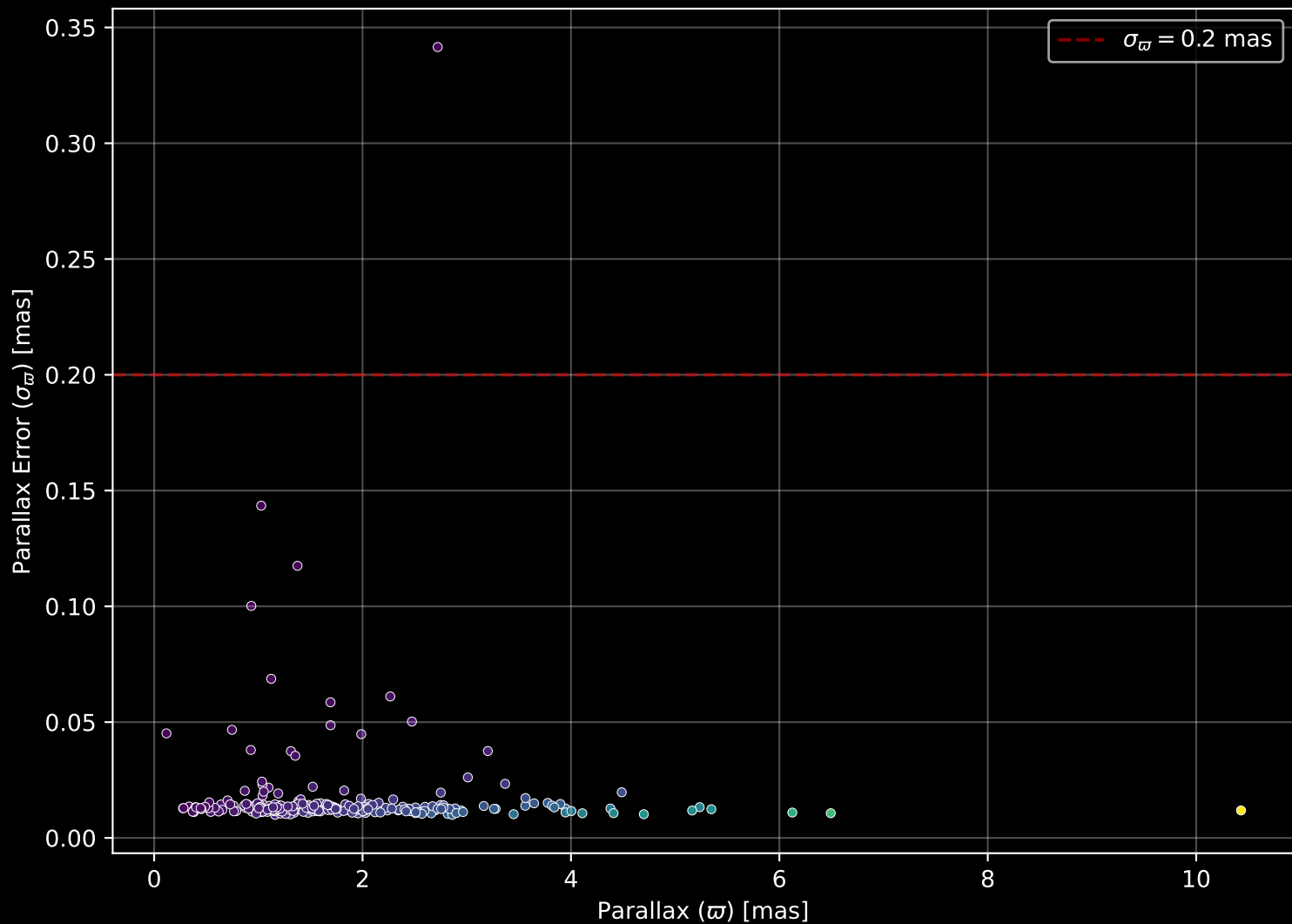
GALAH DR4 Field: [350] Parallax Quality (n= 257)
