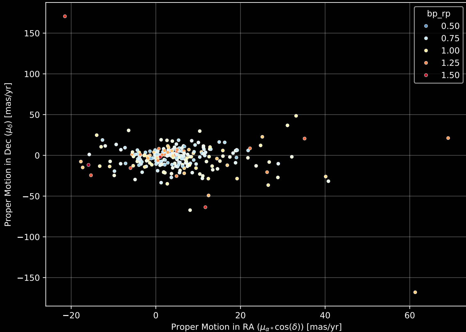
GALAH DR4 Field: [350] Proper Motion Diagram (n= 257)
