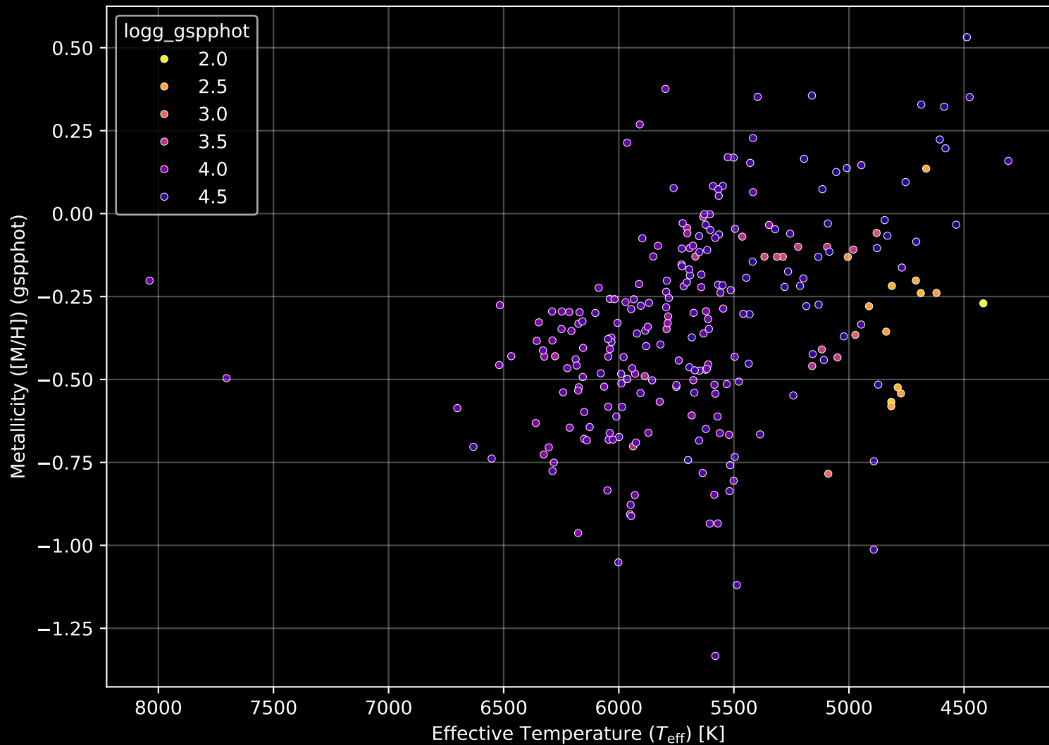
GALAH DR4 Field: [350] Stellar Population Parameters (n= 257)
