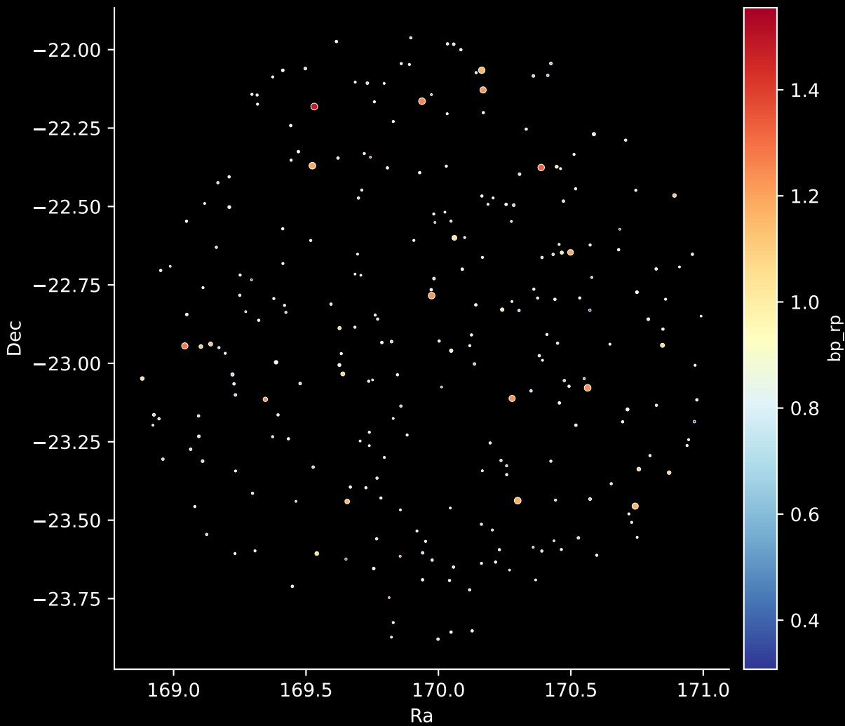
GALAH DR4 Field: [350] Stars: 257
